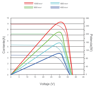
Curvas de Intensidad-Tensión y potencia-tensión (265W)
