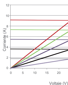
Curvas de corriente-voltaje y alimentación/voltaje (275W)
