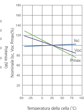
Dipendenza dalla Temperatura di Isc, Voc, Pmax
