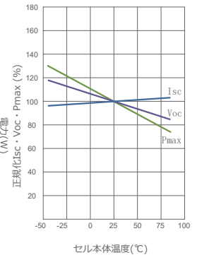
Isc・Voc・Pmaxの温度依存性
