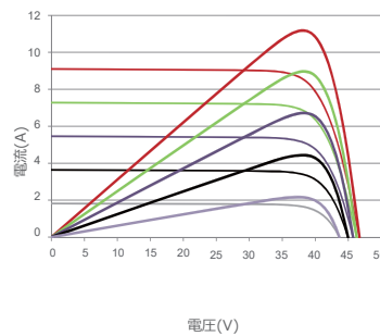
電流電圧・電力電圧特性曲線 (335W)
