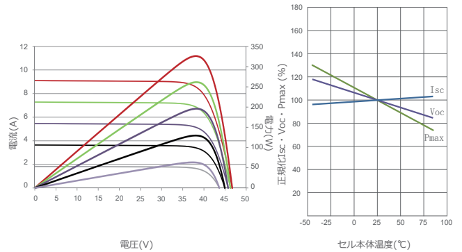
電流電圧・電力電圧特性曲線 (335W)
