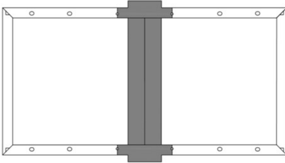
図4：NEXボルト固定方法(4点止め)
