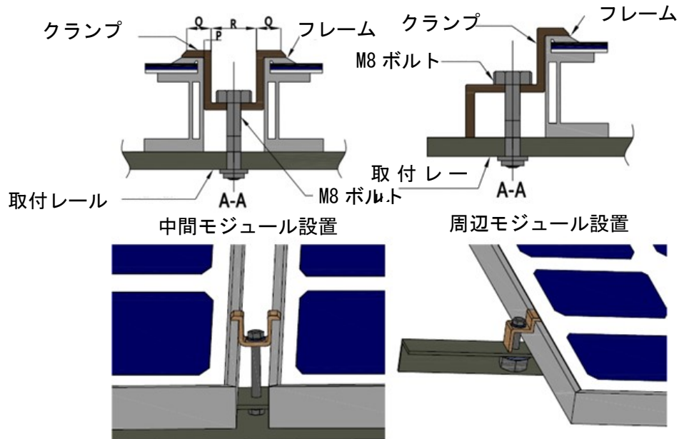
図5：クランプ固定方式
