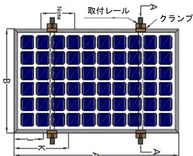
図6：クランプ固定方式（長辺）
