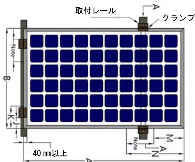
図8：クランプ固定方式(長辺・短辺)
