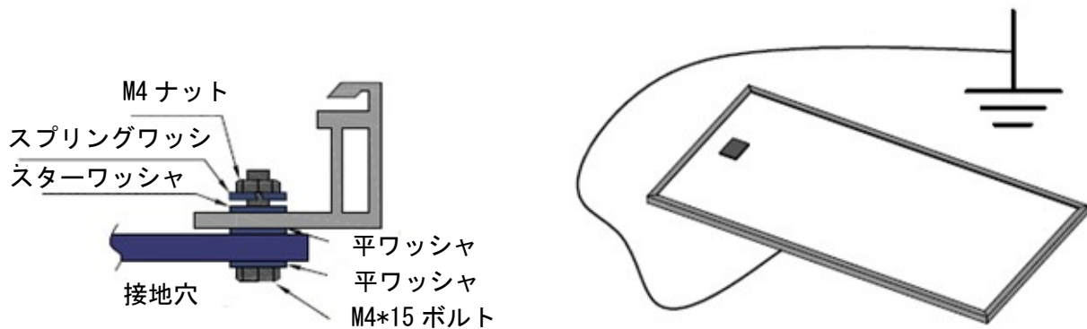
図9: モジュールの接地方法
