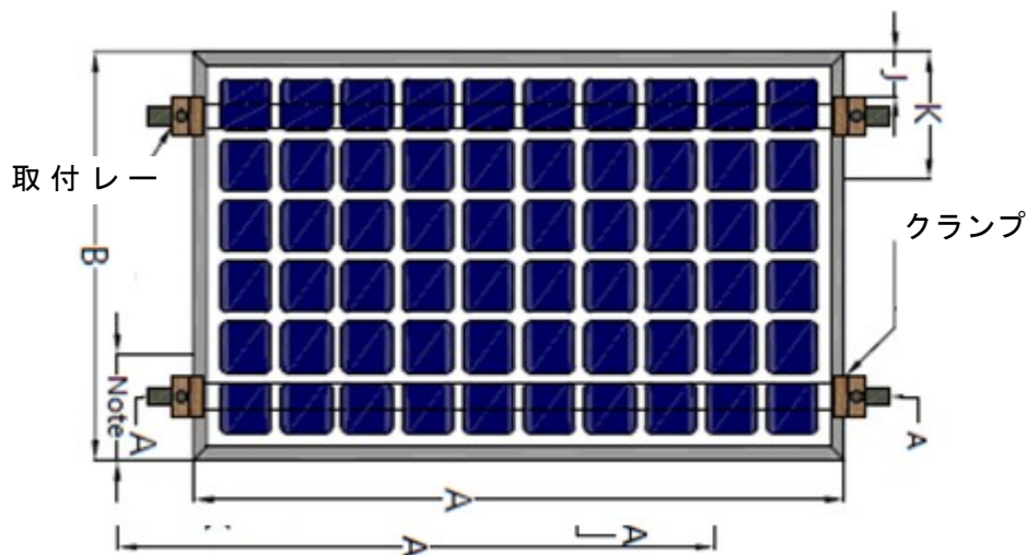
図7：クランプ固定方式(短 辺)
