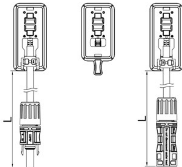
図10(2)：ハーフカットセルモジュール/SWAN両面発電モジュールの端子ボックスの例
