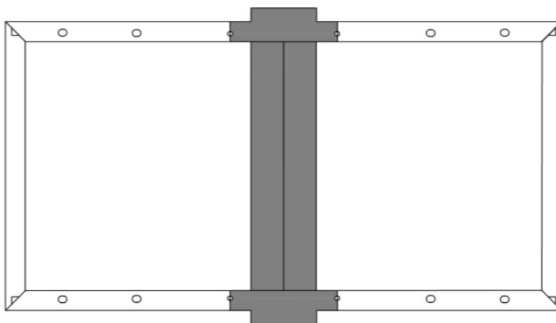
图 5：螺丝固定的方法（4个NEXTracker安装孔）
