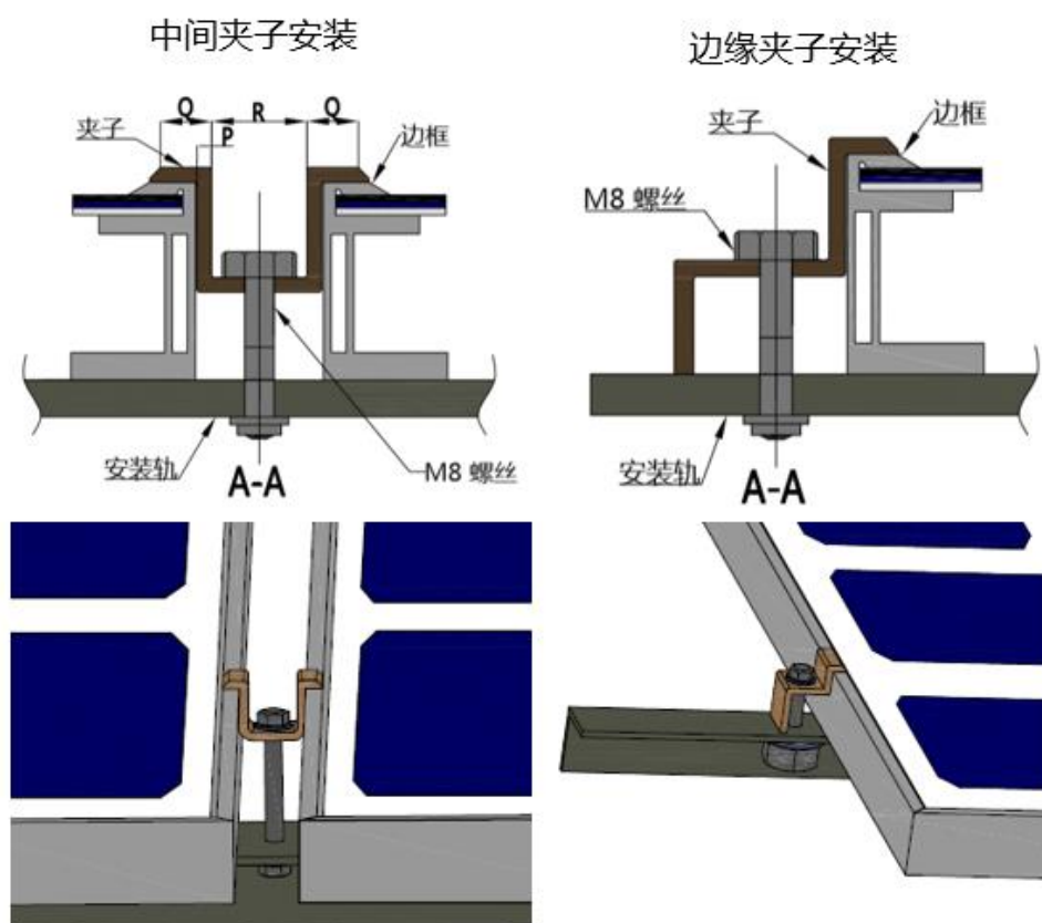
图4：双玻（有框）组件夹子安装方式
