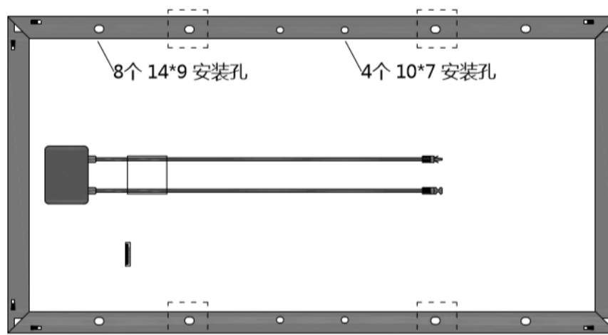
图3：螺丝固定的方法 (4个安装孔)
