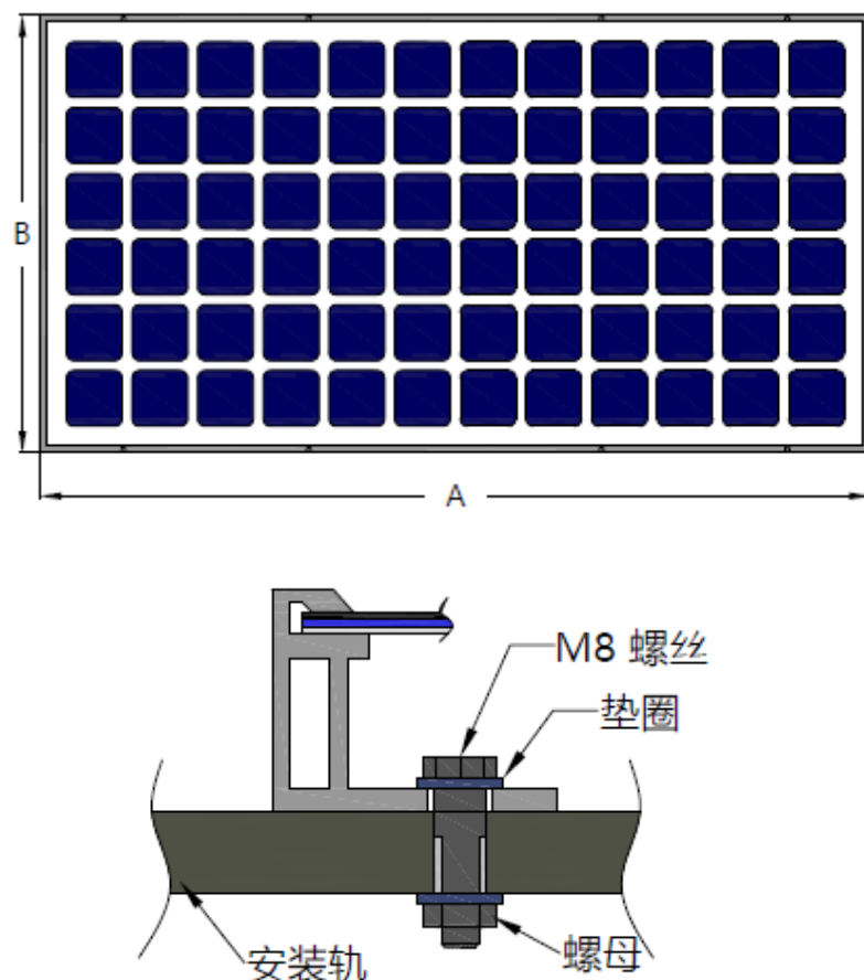
图2：双玻（有框）组件螺丝安装方式
