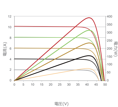
I-V 特性曲線 (390W)
