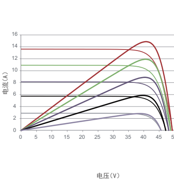
电流电压及功率电压曲线(540W)
