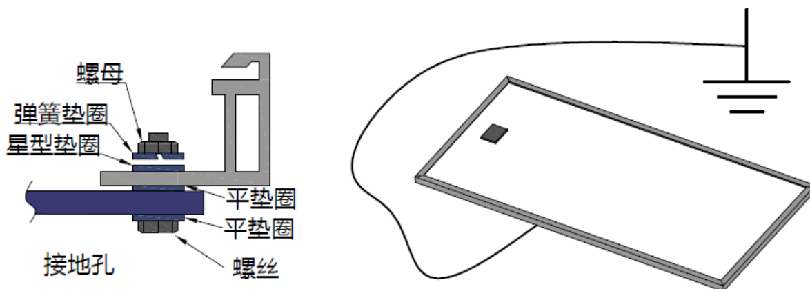
图11：接地图
